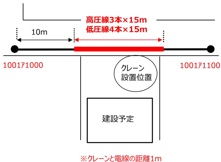
平面図_記載例① 建物建築等クレーン使用時
